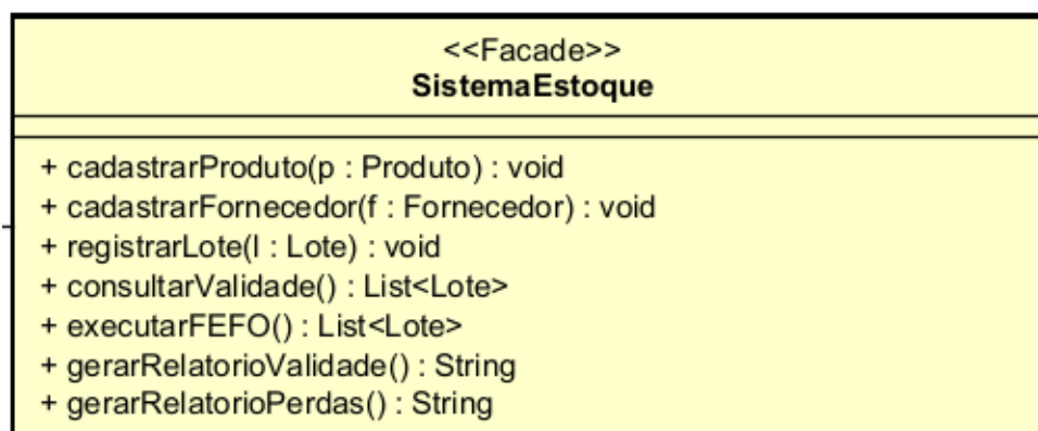
Figura 9: Diagrama:Facade
