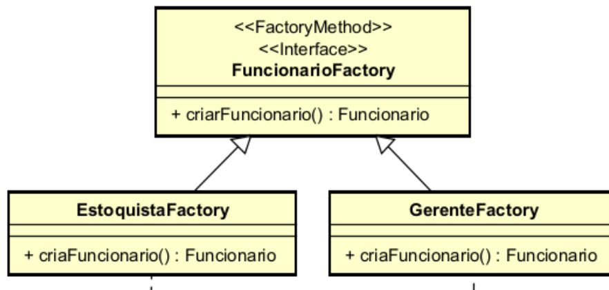
Figura 7: Diagrama:FuncionarioFactory
